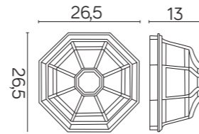
K 3012/P SZ E27 max 60W
