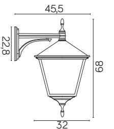
K 3012/1/BD KW E27 max 100W
