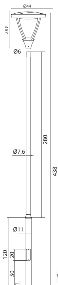
MLS LB-H4400 LED 45 W Strumień świetlny: 3700 lm / Luminous flux (słup z głowicą / pole with head)
