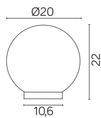
G 200 Z E27 max 60W
