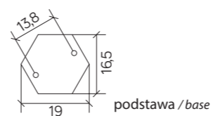
K 5002/3/H E27 max 60W
