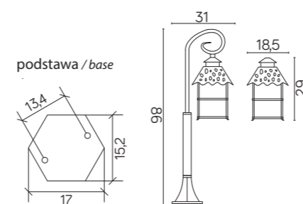
K 5002/3/Z E27 max 60W
