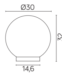
G 300 Z E27 max 100W
