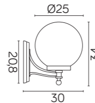
K 3012/1/K 250 OP K 3012/1/K 250 FU E27 max 60W
