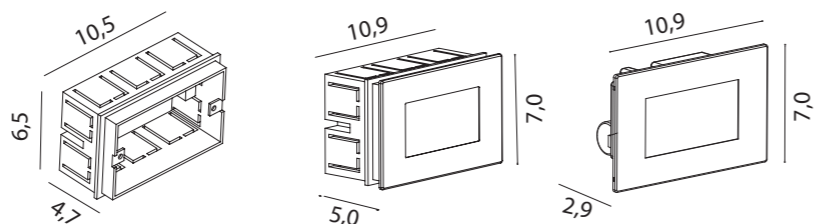
MG01 LED, 2,5 W Strumień świetlny: 195 lm / Luminous flux
