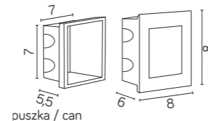
F 04 12 x LED, 1,5 W Strumień świetlny: 64 lm / Luminous flux
