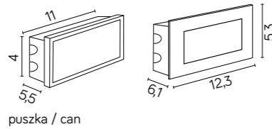
E 04 12 x LED, 1,5 W Strumień świetlny: 64 lm / Luminous flux
