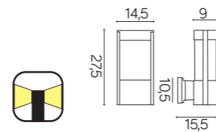
TY 0651 BL E27 max 60W
