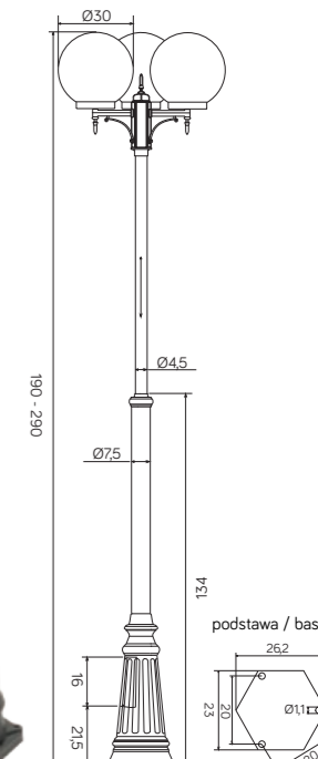
OGMWN 3 300 OP E27 3 × max 100 W
