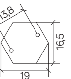
K 5002/1/KPO OP K 5002/1/KPO FU E27 max 60W
