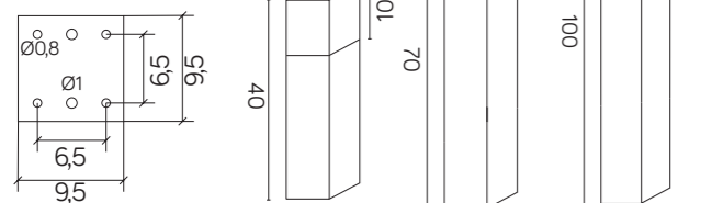
CB-MAX 400 AL E27 max 20W
