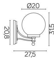
K 3012/1/K 200 OP K 3012/1/K 200 FU E27 max 60W
