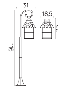
K 5002/2/Z E27 max 60W
