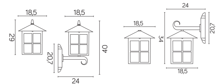
K 3012/1/KW E27 max 60W
