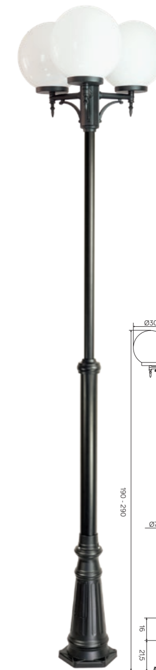
OGMWN 3 300 OP E27 3 × max 100 W
