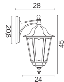
K 3012/1/D E27 max 60W
