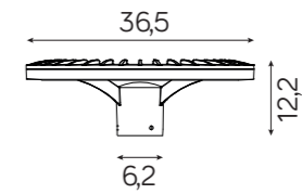
STR-HEAD LED, 44 W Strumień świetlny: 3400 lm / Luminous flux
