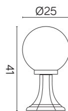
K 4011/1/K 250 OP K 4011/1/K 250 FU E27 max 60W
