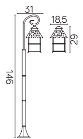
K 5002/1/Z E27 max 60W
