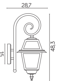
K 3012/1/N E27 max 60W
