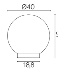
G 400 Z E27 max 100W
