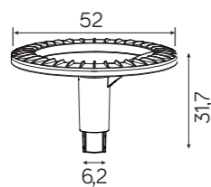
STRMAX-HEAD LED, 60 W Strumień świetlny: 4500 lm / Luminous flux
