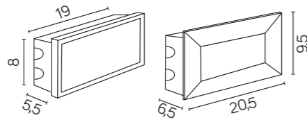
C 04 56 x LED, 3,5 W Strumień świetlny: 187 lm / Luminous flux
