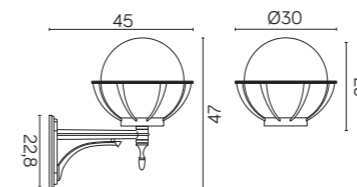
K 3012/1/KPO 250 U FU E27 max 60W
