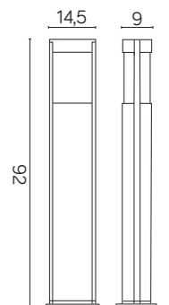
TO 3902-H 919 BL E27 max 60W
